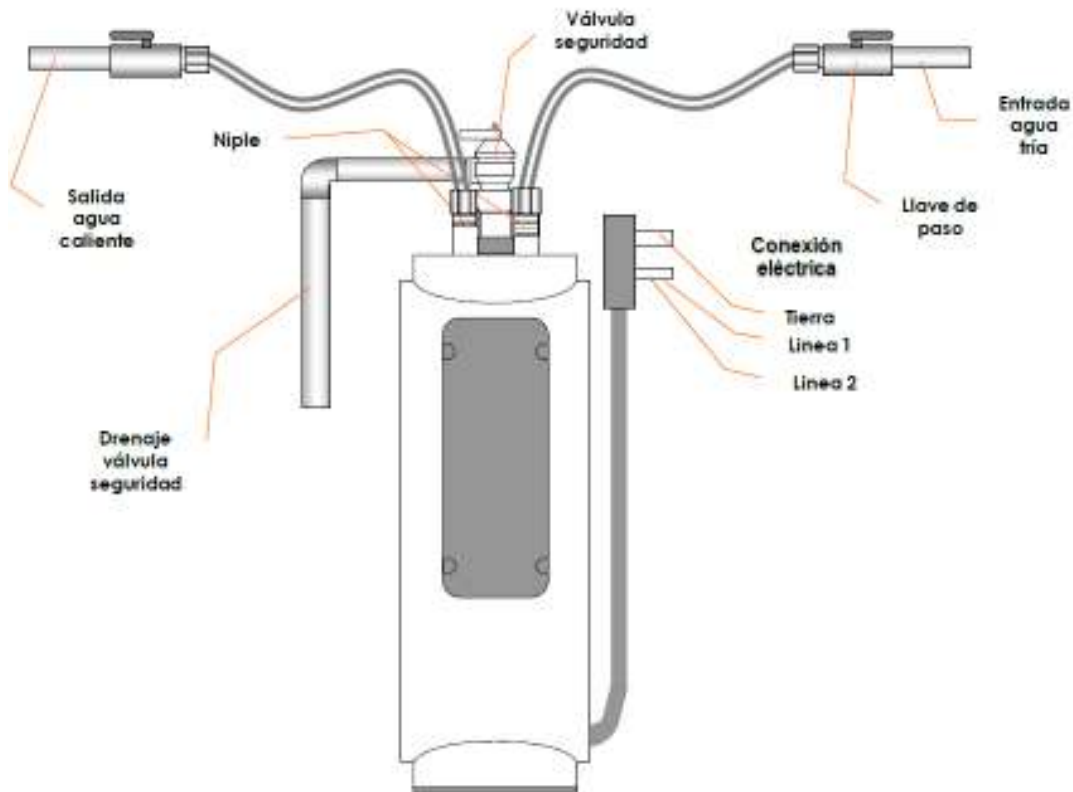
Figura N° 2 Conexión al Sistema de Agua
